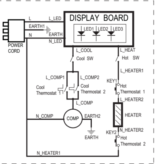
Mẫu máy có ngăn làm lạnh (EQALF01TXWV)
